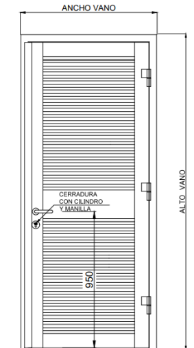
VISTA EXTERIOR
